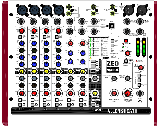
ZED-10FX MIXER
